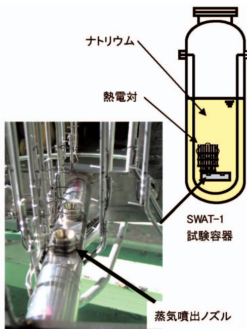
図 1 フリージェット試験用水蒸気ジェット噴出管
