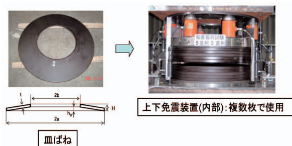
図2 上下免震試験装置全体図
