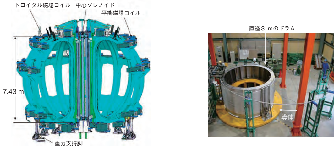
図 3-13 超伝導コイルの組立図と平衡磁場コイル導体の製作状況 欧州はトロイダル磁場コイル(18個)を、日本は平衡磁場コイル(6個)と中心ソレノイド(4モジュール)を調達します。右の写真は、那珂核融合研究所の導体製作棟における平衡磁場コイル用超伝導導体製作の様子です。
