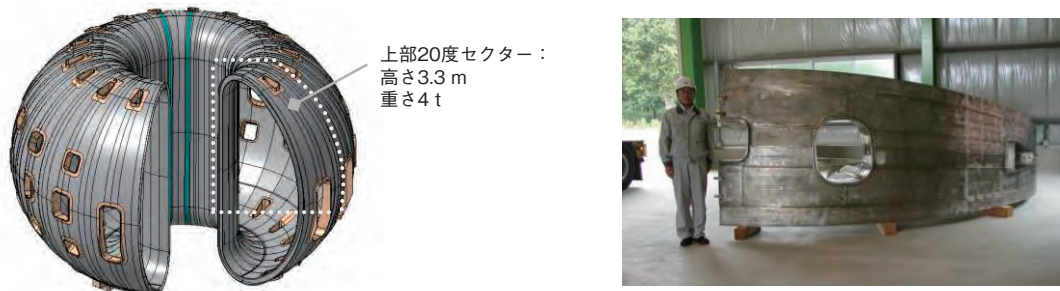
図 3-14 真空容器の組立図と試作試験体 真空容器の組立図に示される上部20度セクターの試作試験が完了し、実機の製作が工場で開始されるとともに、試験体が那珂核融合研究所の真空容器組立棟に搬入されました。
