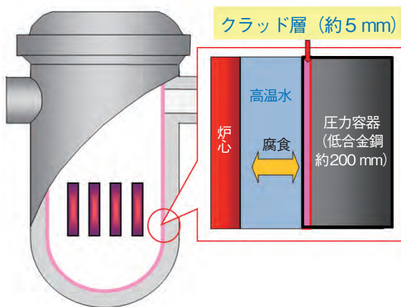
図5-8 压力容器とクラッド層
