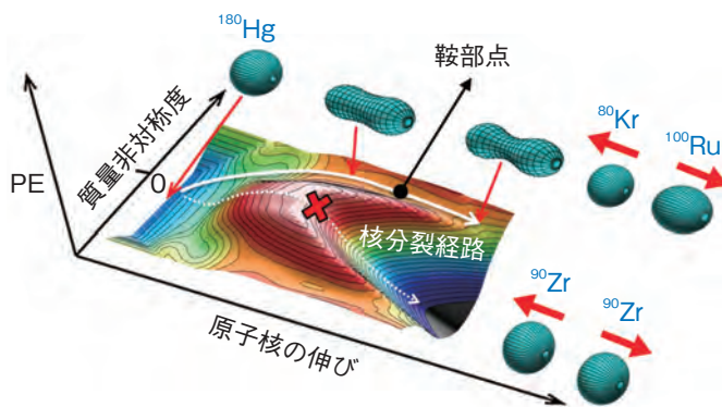
図 6-8 ^{180}\text{Hg} の核分裂経路
