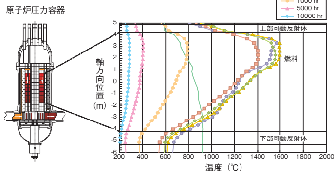
図8-3 炉容器冷却設備 事故後の炉心の残留熱は、空気自然対流やふく射によって原子炉压力容器外側から炉容器冷却設備の冷却パネルへ移行し、冷却パネル内を温度差による自然循環で流れる空気によって大気へ放散されます。電力及び動的機器を使用しない受動的な設備です。
