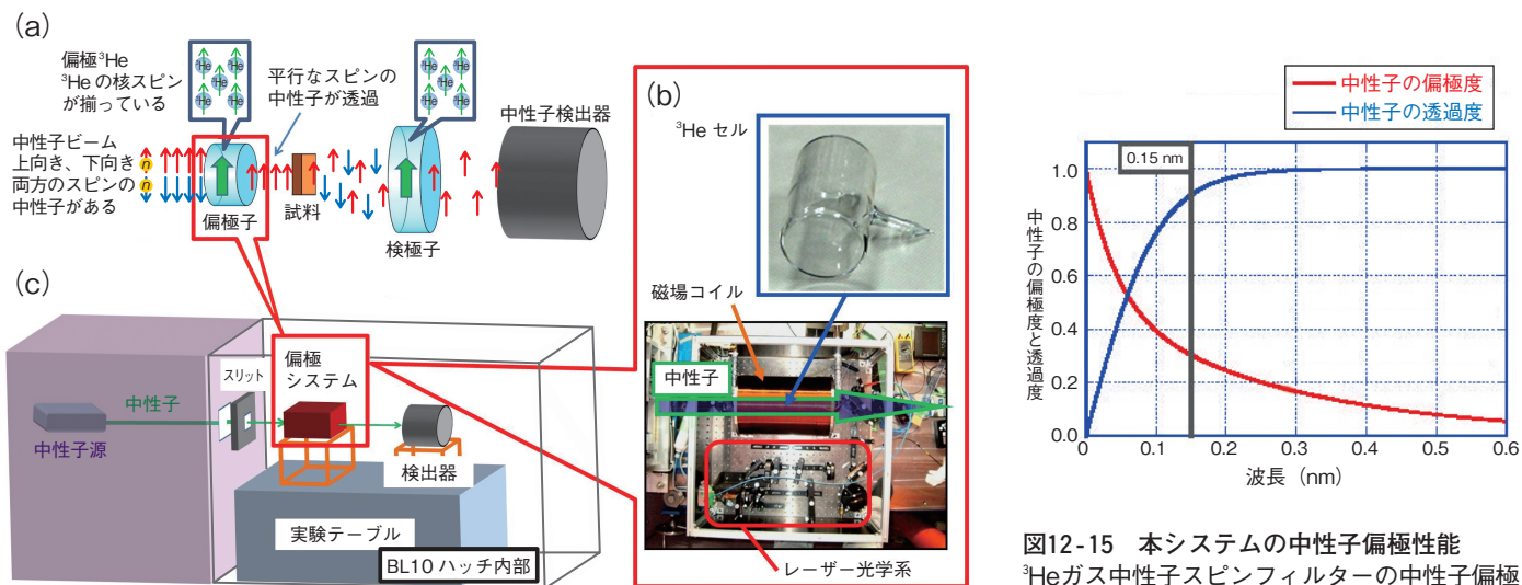
図12-14 偏極 3 He中性子スピンフィルターの概要と評価実験のセットアップ (a) スピンフィルターの概要です。 3 He核スピンと平行なスピンの中性子を選択的に透過させるので中性子ビームの偏極、散乱中性子の検極に役立ちます。 (b) システムの内部の写真です。内部には 3 Heガスセルのほか、レーザー光学系と磁場環境が組み込んであります。 (c) 評価実験のセットアップの様子です。図のようにビーム軸上にシステムを設置し、 3 Heガスの偏極前後の中性子透過率を測定しました。
