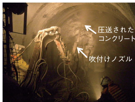
図 2-23 坑道壁面への吹付け状況
