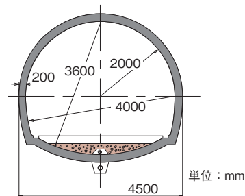
図 2-22 調査坑道の断面図
