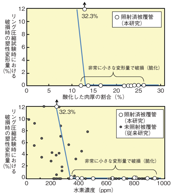
図5-5 冷却材喪失模擬実験に供した被覆管に対するリング圧縮試験の結果 酸化量と水素吸収量が一定量を超えると、非常に小さな変形量で破損します。冷却材喪失模擬実験ではいずれの照射済被覆管も破損しませんが、水素濃度の低いひとつを除き、リング圧縮試験では「脆化した」と判断されます。
