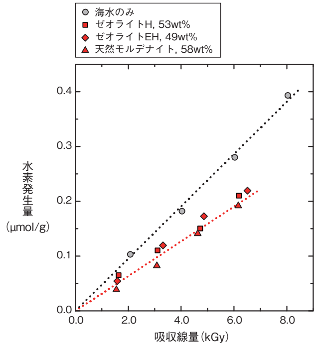
図1-49 ゼオライトと海水との混合物からの水素発生量 ゼオライトと海水との混合物に 60 Coからのγ線を照射し、水素発生量と吸収線量との関係を測定しました。
