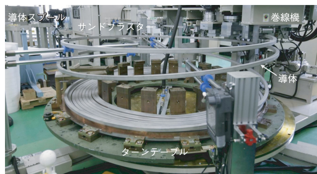
図 4-16 中心ソレノイドの製作状況
