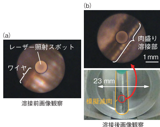
図 13-2 管内壁への肉盛り溶接試験 (a) レーザー照射スポットと溶接ワイヤ送給位置の一致が画像観察できます。(b) 幅約 1 mm、高さ約 0.2 mm 直線状に肉盛り溶接することに成功しました。母材より侵食に強い材料を充てんとすると、次の減肉進展を抑制可能です。
