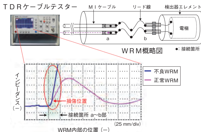
TDR法による特性インピーダンス波形観測
