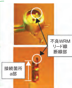
不良WRMリード線断線部
