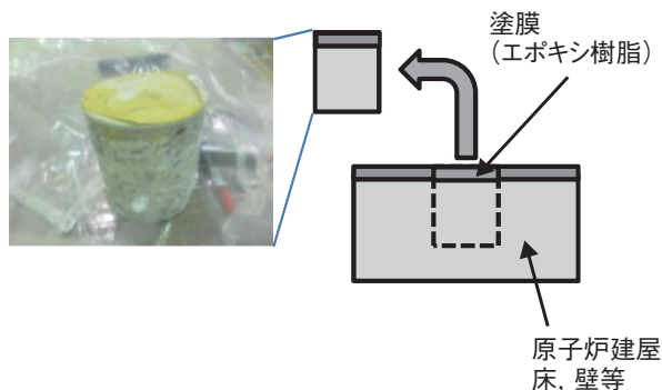
図1-45 コンクリートコアサンプルの外観 1F 原子炉建屋の床、壁等から採取された直径約 10 cm のコンクリートコアサンプルを分析しました。
