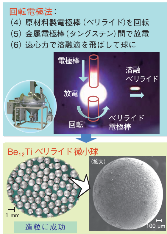
図4-7 回転電極法による微小球製造 プラズマ焼結製ベリライド電極棒を用いて、回転電極法によって、直径約1 mmのベリライド微小球製造に世界で初めて成功しました。
