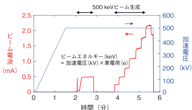
図5-12 500 keV 大電流電子ビーム生成試験
