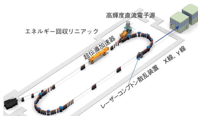
図5-13 エネルギー回収リニアック \gamma 線発生装置
