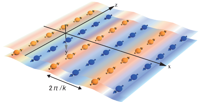
図3-3 金属表面に生じる磁気パターン
