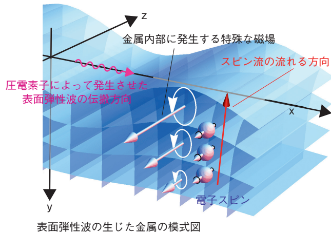
図3-2 音波によるスピン流生成
