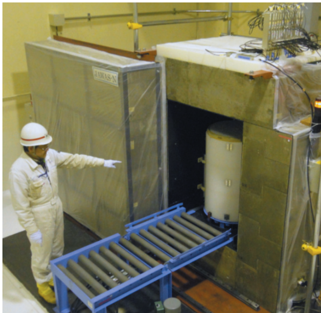
図4-6 人形峠環境技術センター内に構築された非破壊測定装置本体装置(JAWAS-N)の筐体(外観: 縦2 m, 横2 m, 高さ約2.2 m)は、厚さ0.5 mのコンクリートから構成され、その中の空間(縦1 m, 横1 m, 高さ1.2 m)にドラム缶回転台, 中性子発生管, 3 He 検出器が組み込まれたディテクターバンクが収められています(図4-7)。
