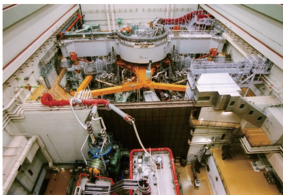
図9-13 JT-60 解体前の本体室
