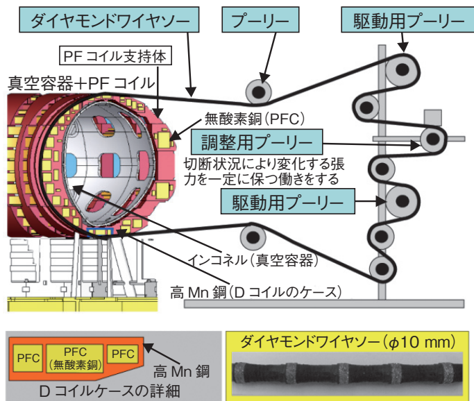
図9-15 ダイヤモンドワイヤソーシステム
