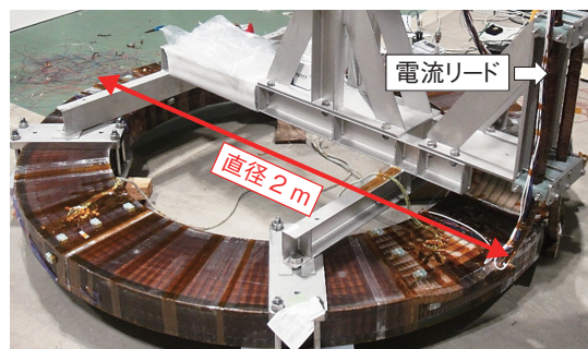
図9-17 CS モデルコイル
