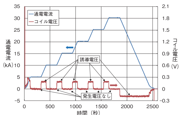
図9-18 CS モデルコイル発生電圧測定
