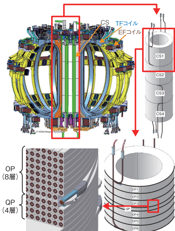
図9-16 JT-60SA 用中心ソレノイド
