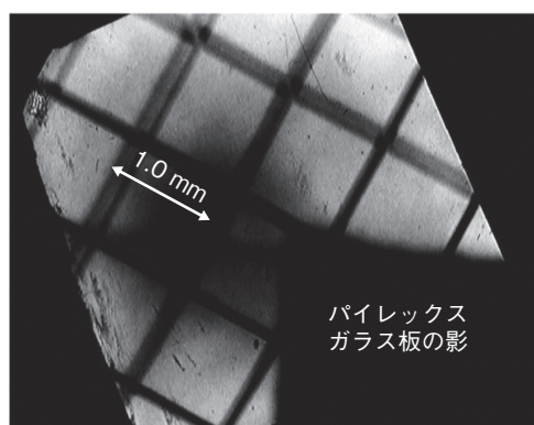
図 5-33 Na を透過した紫外線の照明により取得したメッシュ像
