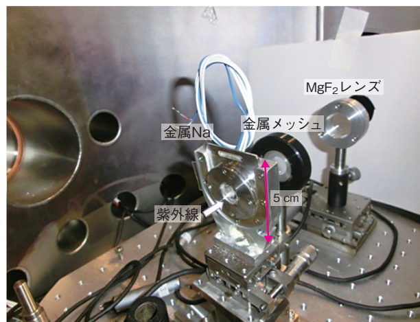
図 5-32 Na サンプルとイメージング装置
