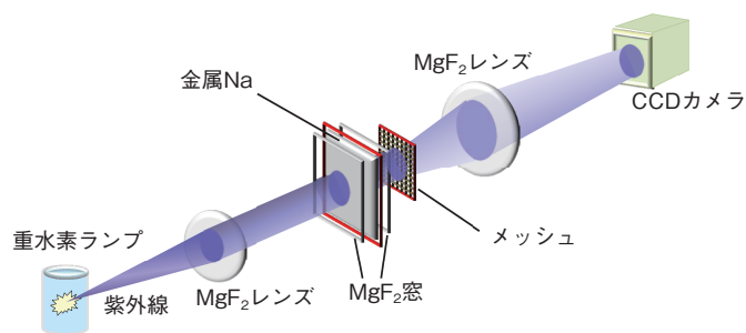
図 5-31 実験配置
