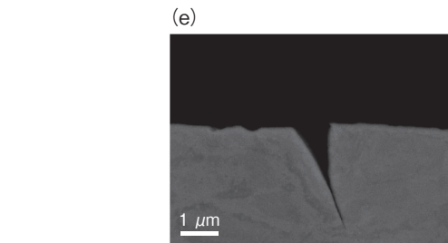
図4-8 リン化合物の濃縮がある場合の粒界腐食形態 (c)、(d)は本モデルによるシミュレーション結果です。リン量が増える領域から粒界腐食幅が狭くなる結果となりました。シミュレーション結果(d)は、腐食試験で見られた複雑形状の腐食形態(e)を模擬できていることが分かりました。
