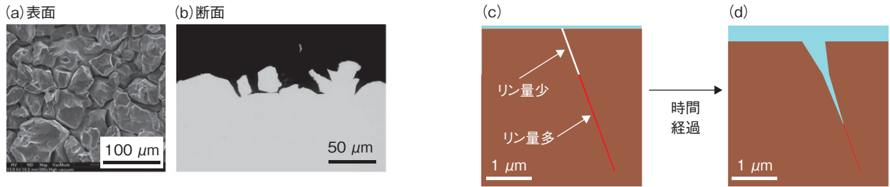
図4-6 硝酸溶液中ステンレス鋼の粒界腐食の例 高温高濃度の硝酸溶液中にあるステンレス鋼は、(a)のように結晶粒間にある粒界が優先的に腐食する粒界腐食が発生します。断面を見ると(b)のような複雑な凹凸形状になっています。
