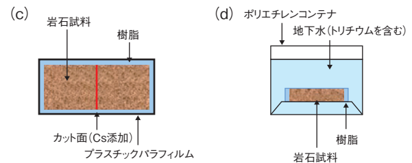
図 8-19 室内拡散試験の概略
