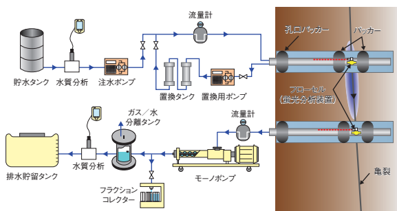
図 8-17 原位置試験装置のシステム
