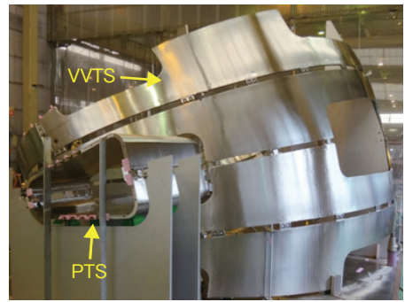
図9-15 VVTSの仮組み 実機製作した10度のVVTSを40度まで仮組みをして、製作寸法が寸法公差以内であることを確認しました。
