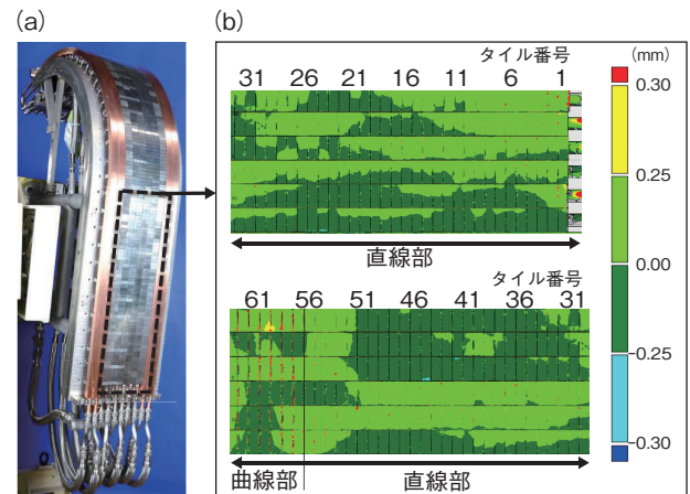
図9-6 フルタンングステンプラズマ対向ユニット（実規模プロトタイプ）の外観と表面の三次元測定結果 (a) 高熱負荷試験架台にプラズマ対向ユニット6本を設置した様子です。(b) 組み立て後のタンングステンタイルの表面輪郭度の計測結果です。カラーは理論表面と計測値の差を表しており、直線部が \pm 0.3 mmの要求精度内にあることが確認できました。
