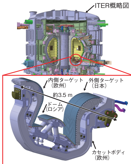
図9-5 ITER ダイバータの構造（カセット構造） ITER ダイバータは、外側ターゲット、内側ターゲット及びドームをカセットボディと呼ばれる筐体に設置したカセット構造となっており、54個のカセットでダイバータを構成します。
