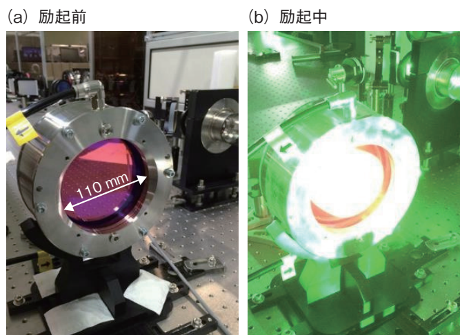
図 5-27 J-KAREN-P でエネルギー増幅に用いる Ti:Sap 結晶 (a) J-KAREN-P では世界最大級である直径 120 mm の Ti:Sap 結晶を水冷用の治具に固定して用います(有効径: 110 mm)。 (b) 強力な緑色の励起レーザーを照射することで、中心の白い部分にエネルギーが蓄えられています。
