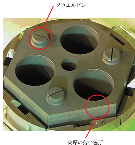
図6-12 制御棒案内ブロックの外観検査 原子炉压力容器内の制御棒案内ブロックは、起動用の中性子源の交換作業の際に取り出されました。東日本大震災後、初めて外観検査を実施、損傷等の異常がないことを確認するとともに、耐震解析結果の妥当性を検証できました。
