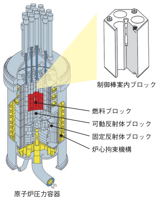
図6-11 HTTRの原子炉压力容器と制御棒案内ブロック HTTRの原子炉压力容器内の構造図と制御棒案内ブロックを示しています。原子炉压力容器内の構造物は、主に黒鉛で構成されており、制御棒案内ブロックのほかに燃料ブロック、可動反射体ブロック、固定反射体ブロック等が設置されています。
