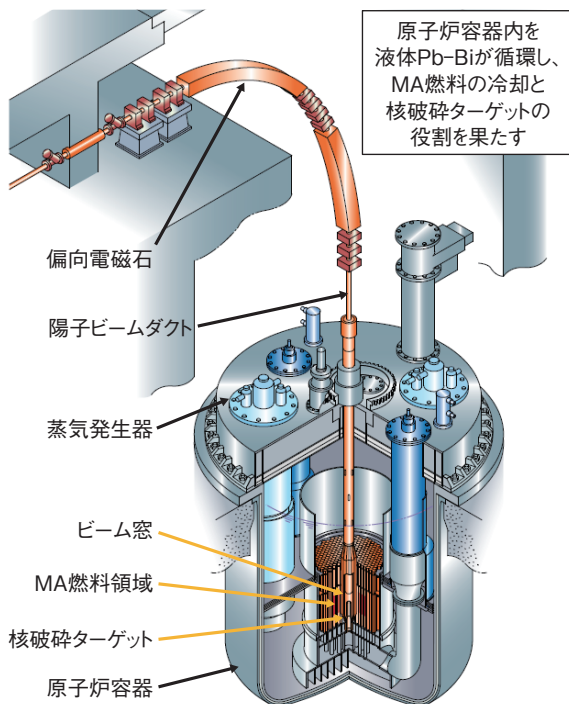
図 4-22 ADS の概念図
