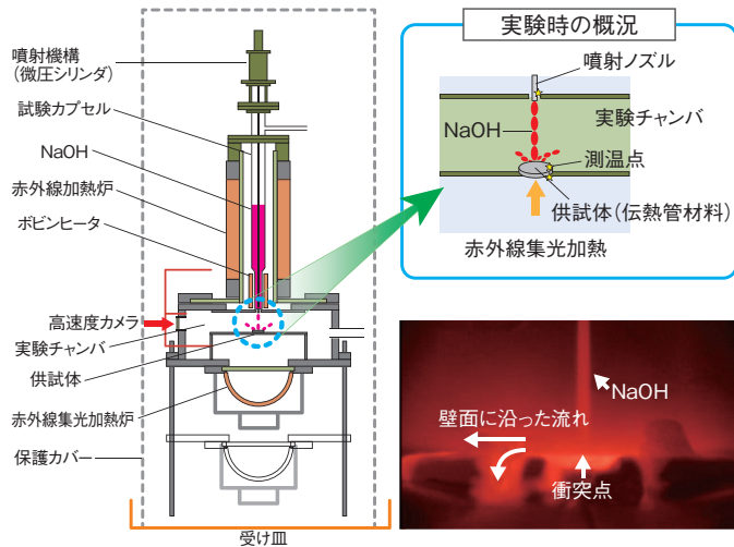
図 7-7 実験装置及び実験状況
