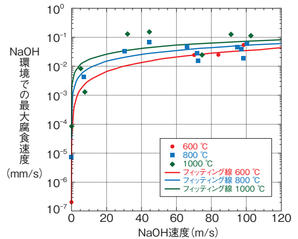
図 7-8 高温 NaOH 環境での腐食速度
