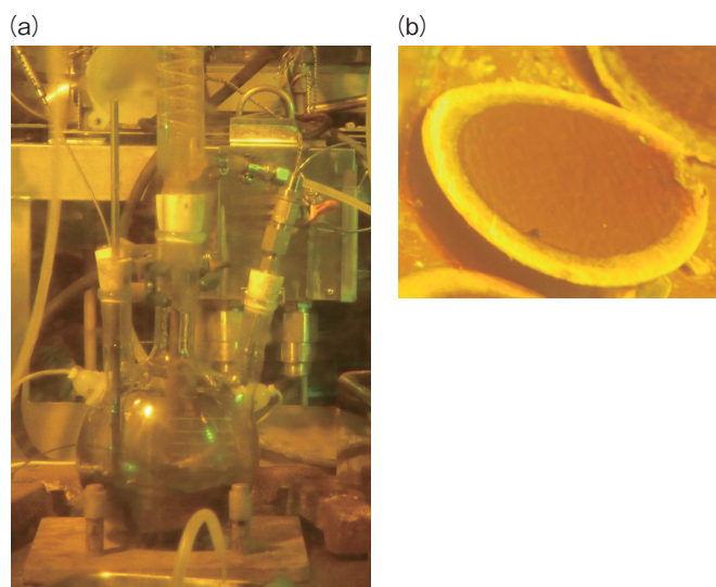
図 8-26 (a) 燃料溶解の様子と (b) ろ過した残渣
