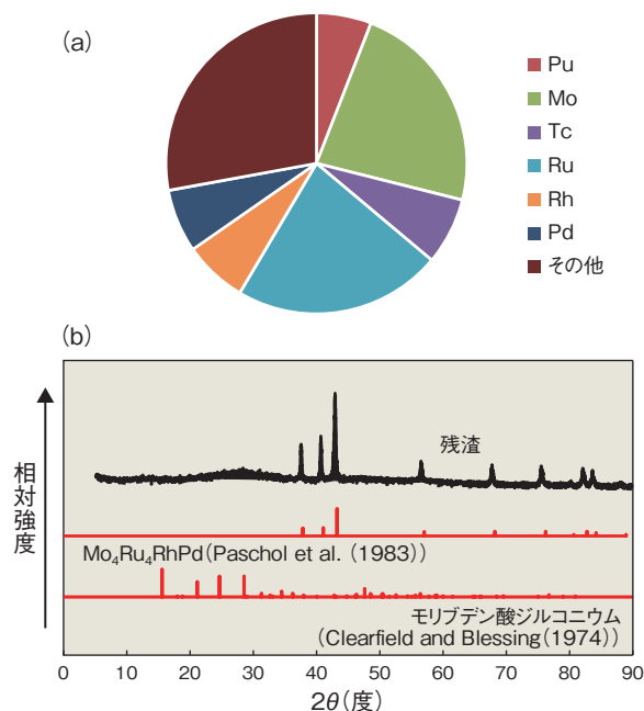
図 8-27 (a) 残渣の化学組成と (b) XRD 分析結果
