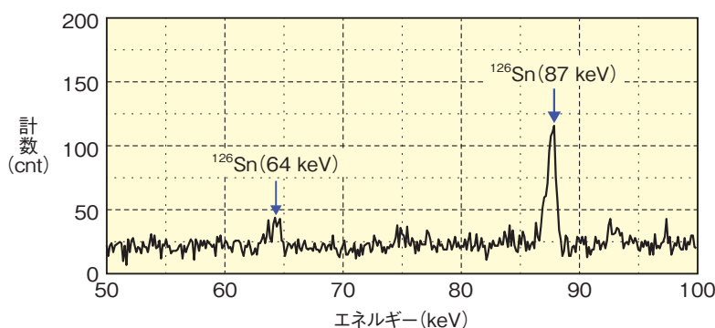
図1-21 Ge-LEPを使用した 126 Sn測定スペクトル 126 Snの壊変時に放出される64 keVと87 keVの2本のγ線がピークとして確認できます。
