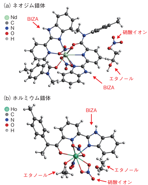
図5-21 ランタノイドと BIZA の錯体の結晶構造 (a) がネオジムと BIZA の錯体構造で、(b) がホルミウムと BIZA の錯体構造です。(a) ではネオジムイオンの左上と右下の空間に、(b) ではホルミウムイオンの上部の空間に BIZA があります。また、空いている空間を埋めるようにエタノール分子や硝酸イオンも存在しています。
