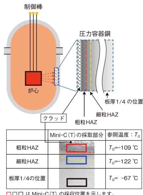
図 2-16 Mini-C(T)を用いたHAZ領域の破壊靱性分布
