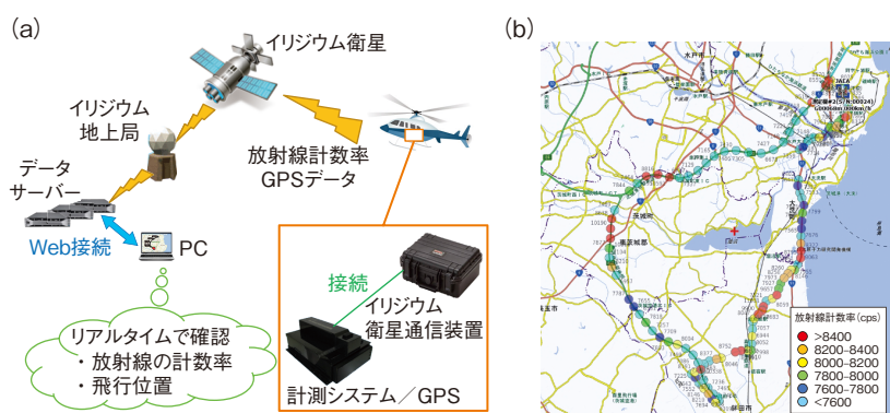
図2-18 リアルタイムに航空機モニタリングデータを共有する通信システム
