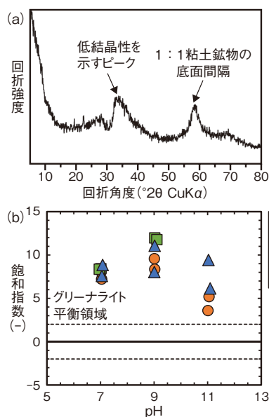
図8-22 Fe(II) と Si の反応試料の固相特性と溶液化学 (a) は共沈生成物の典型的な X 線回折分析結果で、二つのブロードなピークは非晶質で乱層構造の粘土鉱物の生成を示唆しています。(b) は熱力学計算との比較から全ての試験条件で Fe(II) 粘土鉱物であるグリーンナライトの生成を示唆しています。
