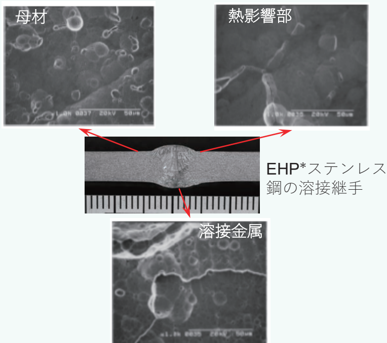
溶接継手断面の沸騰硝酸中腐食試験の結果
