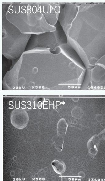
沸騰硝酸中腐食試験の結果
