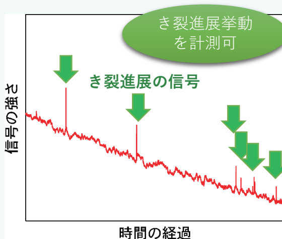
卓上引張試験装置で実施可能
