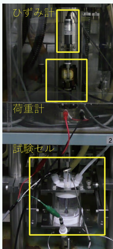
卓上引張試験装置で実施可能
