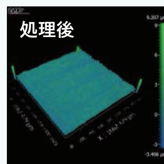
洗浄処理前後の金属表面の凹凸 数 10 \mu\text{m} の凹凸状の汚染物がほとんど剥離
