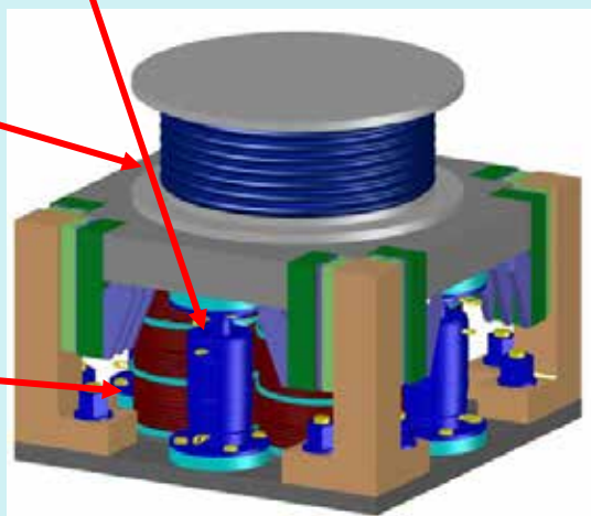
ユニット型3次元免震装置概念図
