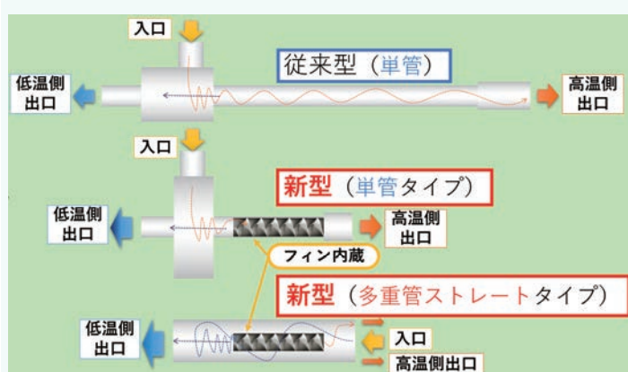
図1 螺旋状フィンを内蔵した新型ボルテックスチューブ
