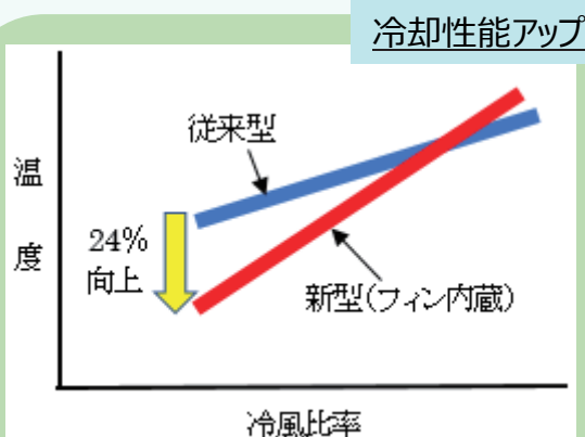
図2 従来型と新型との冷却性能比較
