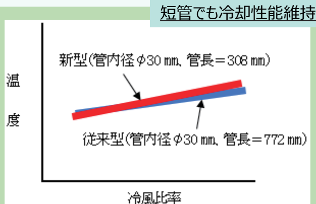
図3 長管と短管との冷却性能比較
